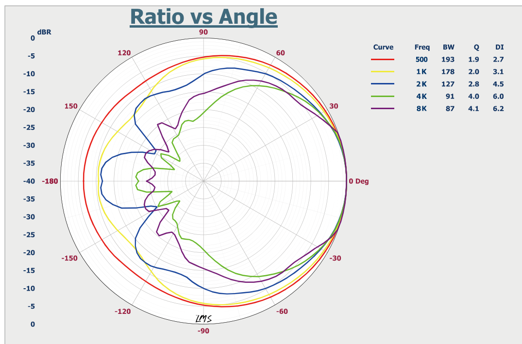
Круговая диграмма направленности громкоговорителя LPA-40MB
